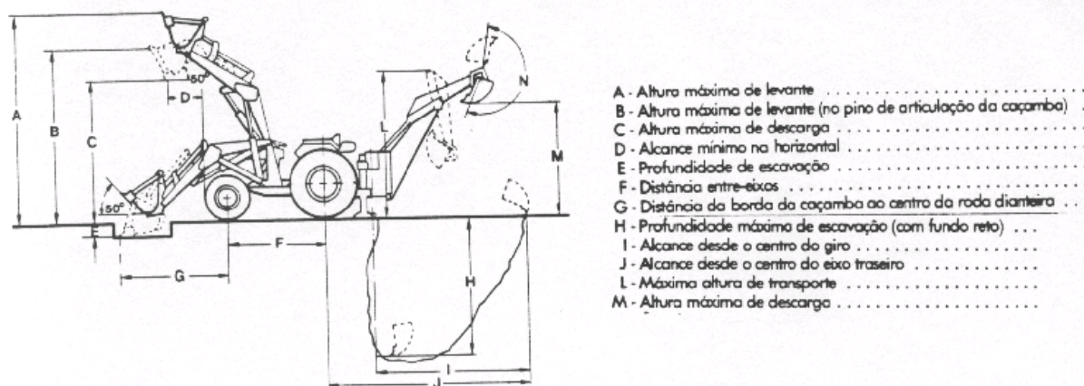
Figura 14 – Retro-escavadora equipada com pá-carregadora.
